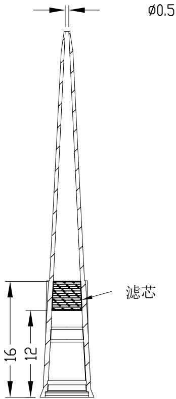
SECTION A-A
